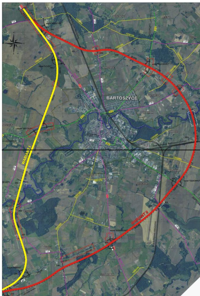
Rysunek nr 1. Przebieg projektowanej obwodnicy Bartoszyce w ciągu drogi krajowej nr 51 w wariacie zachodnim i wschodnim
