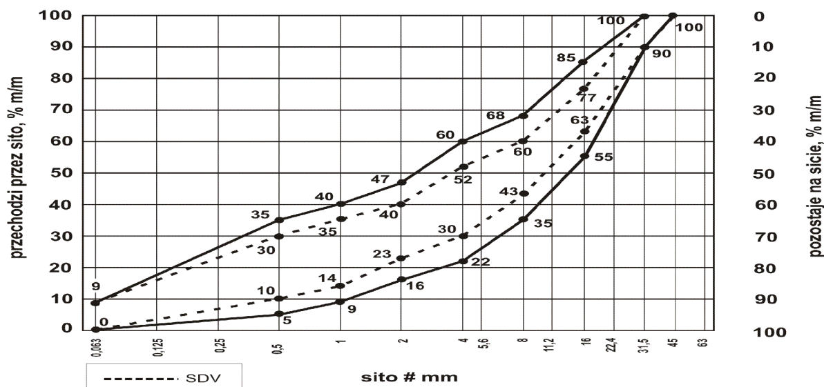
ys. 6.4.4. Uziarnienie mieszanki niezwiązanej 0/31,5 do podbudowy zasadniczej
