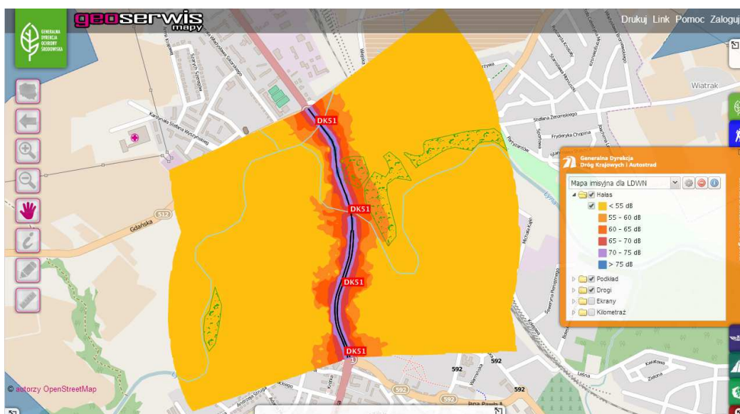
Rycina 10 Mapa emisji dla wskaźnika LDWN przy drodze krajowej DK 51 na terenie miasta Bartoszyce
