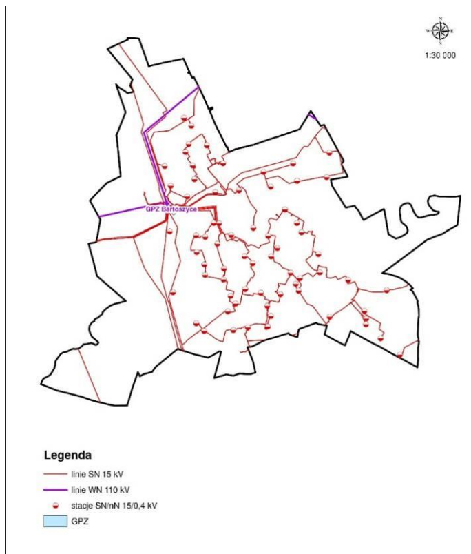
Rysunek 9 Schemat sieci elektroenergetycznej w Bartoszycach
