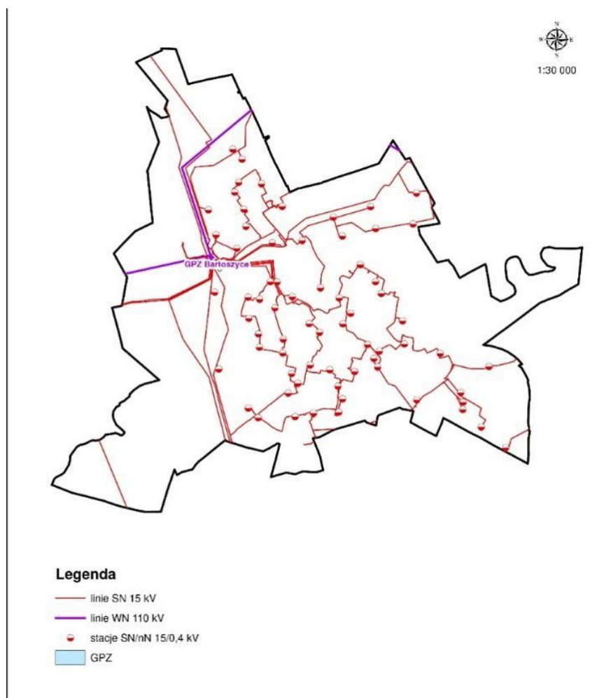
Rysunek 9 Schemat sieci elektroenergetycznej w Bartoszycach
